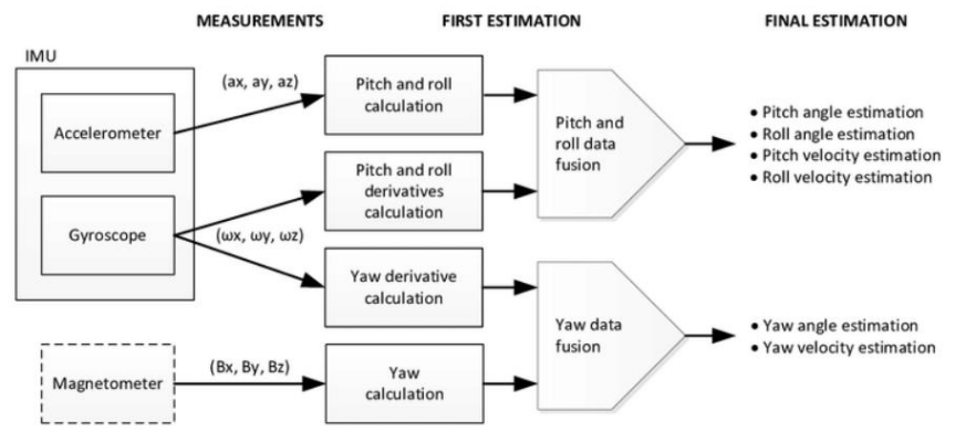
Gambar 7 Blok Diagram Prinsip Kerja IMU (Sumber: https://repository.its.ac.id/ )
